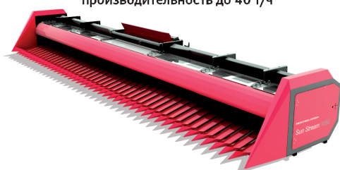
ЖАТКА ДЛЯ УБОРКИ ПОДСОЛНЕЧНИКА SUN STREAM 780/920 ширина захвата до 9,2 м производительность до 7,3 т/ч
