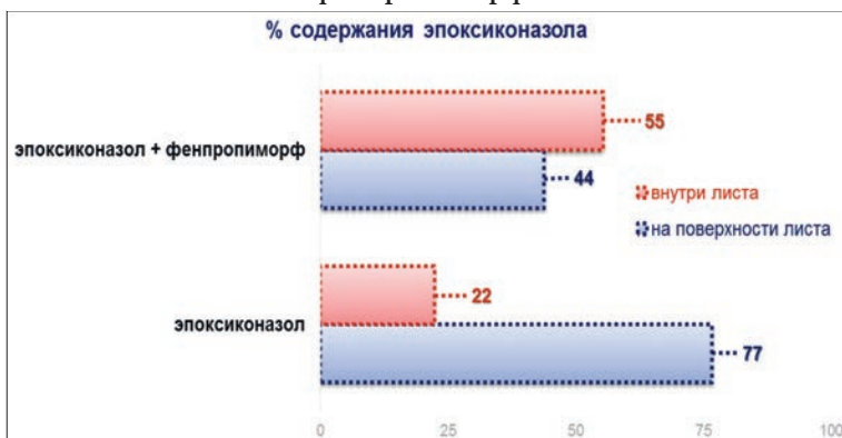
Рис. 2. Распределение эпоксиконазола при применении отдельно и при совместном использовании с фенпропиморфом
