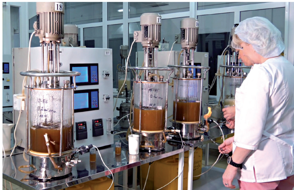
В ферментёрах производится глубинное культивирование бактерий
