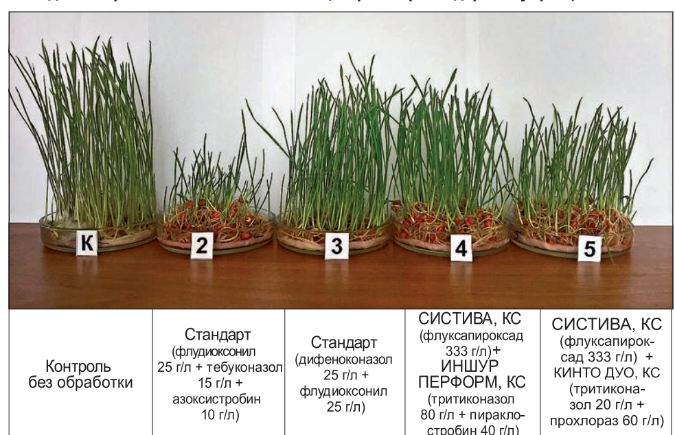
Рис. 2. Развитие озимой пшеницы на 10-й день после обработки, сорт Васса, данные филиала ФГБУ «Россельхозцентр» по Краснодарскому краю, 2016 г.
