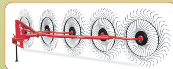
Грабли ворошилки 3,3 м, 6,3 м (Турция, Польша)
